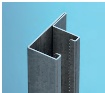
Zahnschiene innen, B 70 x T 37 mm 901201 (WP W03-02)
